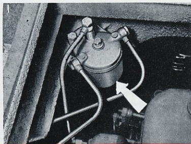
00-14 - Emplacement filtre combustible sur cabine avancée.
