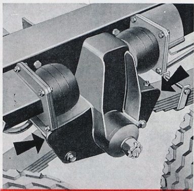
06-8 - Graissage patins de ressorts AR. et lames sur balancier - châssis 6 x 2
