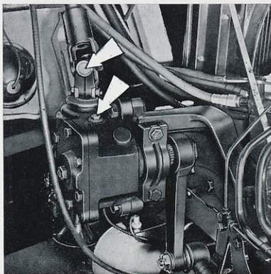
05-4 - Remplissage des boîtiers de direction et graissage des cadrans de colonne de direction (cabine bascul.)
