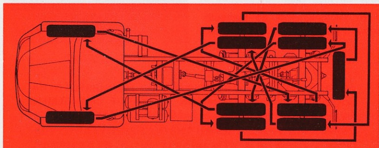
06-9 - Schéma de permutation des pneus (châssis 6 x 4).
