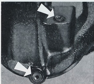
03-1 - Remplissage et vidange sur Pont AR P. 386.
