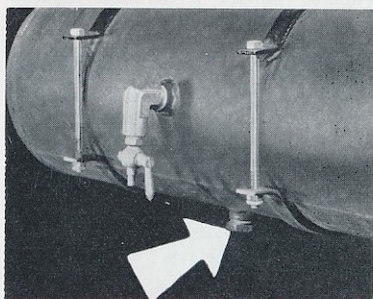
08-19 - Entretien Purge des Réservoirs d'air.
