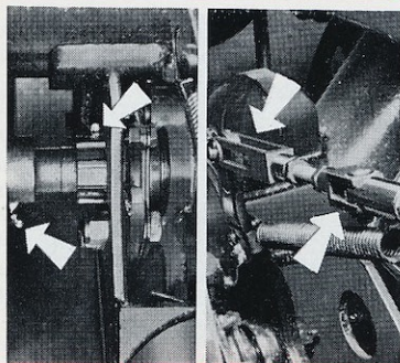
08-11 - Axe de came de frein huilage chape et réglage sur Pont AR N° 2.
