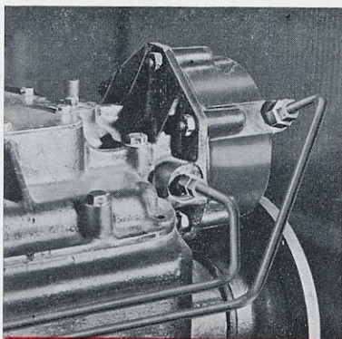
08-18 - Entretien de cylindre de Cde de réducteur sur boîte B. 181.
