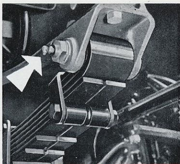
06-1 - Axe avant de ressort AV.
