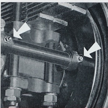
08-2 - Graissage paliers d'arbres à cames.
