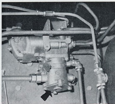
08-13 - Entretien de la centrale de freinage.
