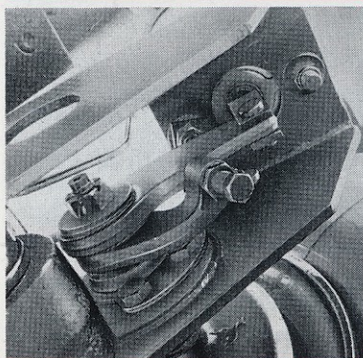
08-9 - Graissage chape Ressort et réglage sur levier de frein Pont AR N° 1.
