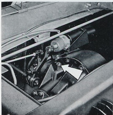
03-2 - Soupape d'aération sur Pont AR P. 386.
