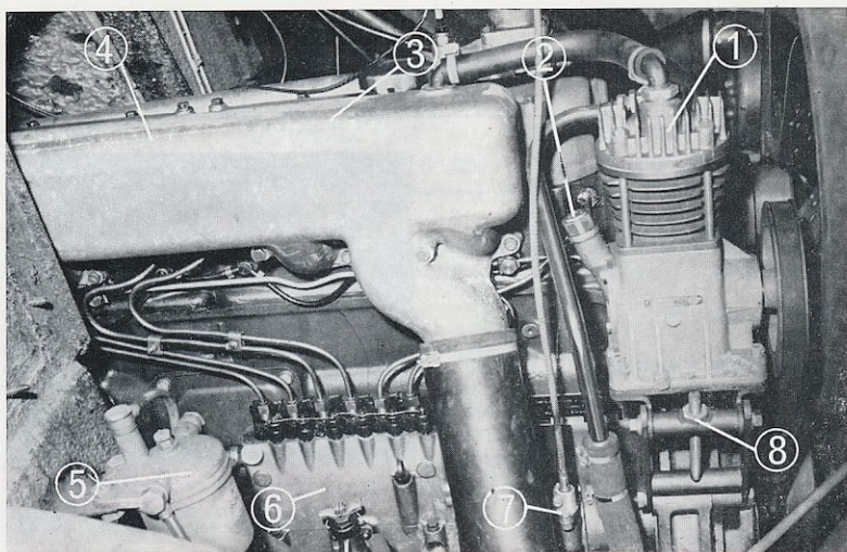
00-3 - Vue d'ensemble moteur capot ouvert sur CSA.
