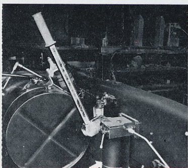
10-7 - Pompe hydraulique pour levage de cabine.
