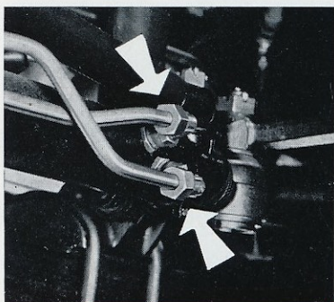
05-8 - Vidange du circuit hydraulique de servo-direction.
