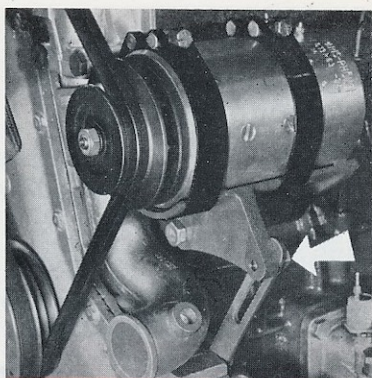
00-24 - Tension de courroie de dynamo (moteur 6 cyl).
