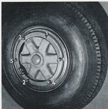
06-10 - Ordre de serrage des roues AV
