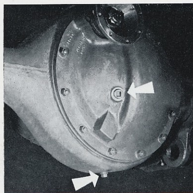
03-3 - Orifice de vidange et niveau sur pont AR n° 1 (chassis 6 x 4).
