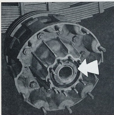
06-13 - Graissage des moyeux AR.
