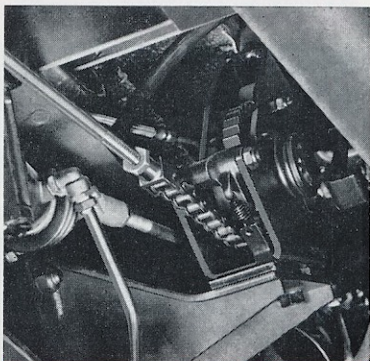
08-3 - Graissage mécanisme de frein à main.
