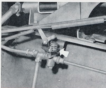
08-17 - Entretien valve de réducteur de vitesses.
