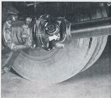
07-4 - Cardan de l'entrée de Pont AR en coulisse. Véhicule 6 x 2.
