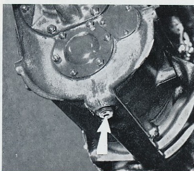
02-2 - Vidange de la boîte de vitesses B 181.
