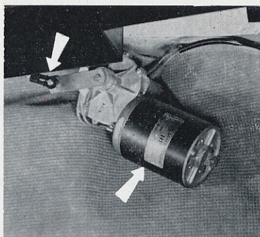
10-1 - Emplacement moteur essuie-glace - CSA.
