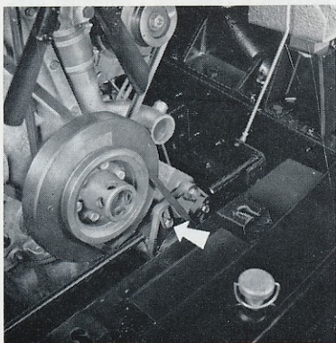
00-25 - Tension de courroie de pompe de servo-direction.
