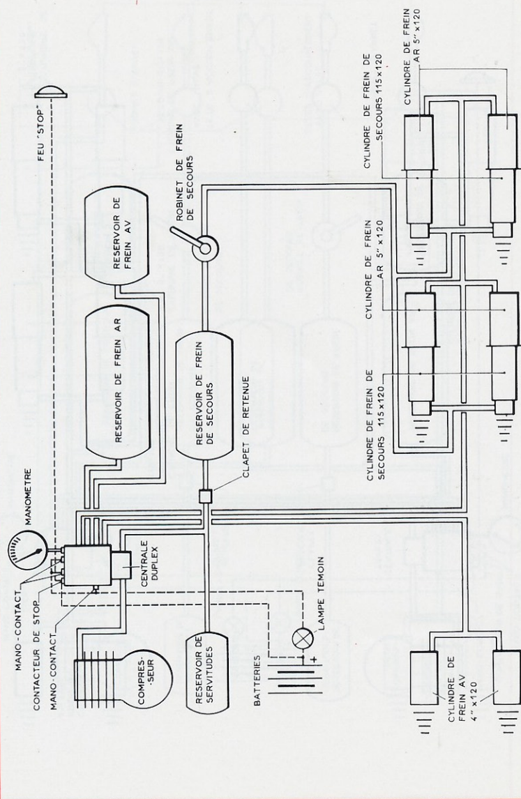
SCHEMA D'INSTALLATION DE FREINAGE (CENTRALE DUPLEX) CHASSIS IZOARD PORTEUR 6 x 2 - 6 x 4
