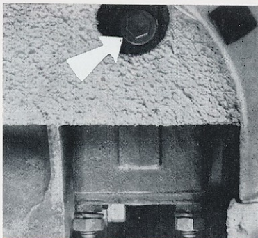
05-2 - Bouchon de remplissage de boîtier de direction (C. A.).
