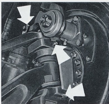
04-1 - Graissage axes de pivot - essieu E 236.
