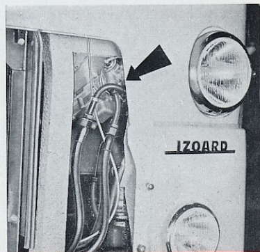
08-15 - Entretien du robinet de freinage. Commande au pied sur C.A. basculante.
