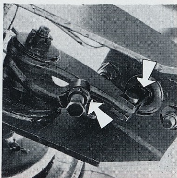
08-12 - Graissage chape et ressort et réglage du levier sur Pont AR N° 2.
