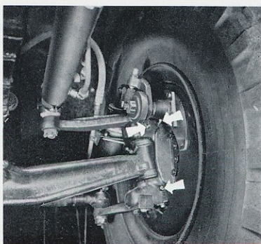
04-3 - Graissage axes de pivot - essieu E 252.
