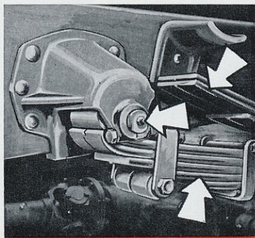
06-3 - Axe avant de ressort AR.
