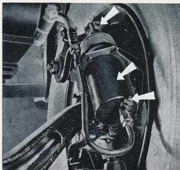
08-5 - Graissage chapes sur levier de frein AV et réglage de frein (E 251).
