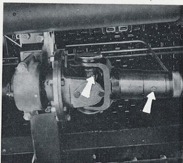
07-1 - Palier intermédiaire de transmission et coulisse de cardan
