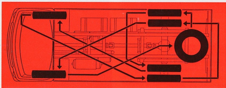
06-8 - Schéma de permutation des pneus (châssis 4 x 2).
