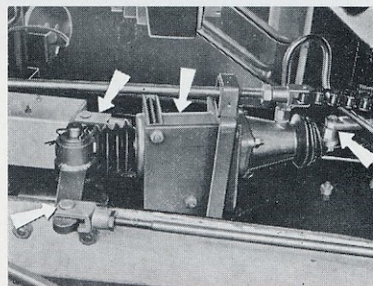
01-3 - Chapes sur cylindre d'assistance de débrayage (servo-débrayage)
