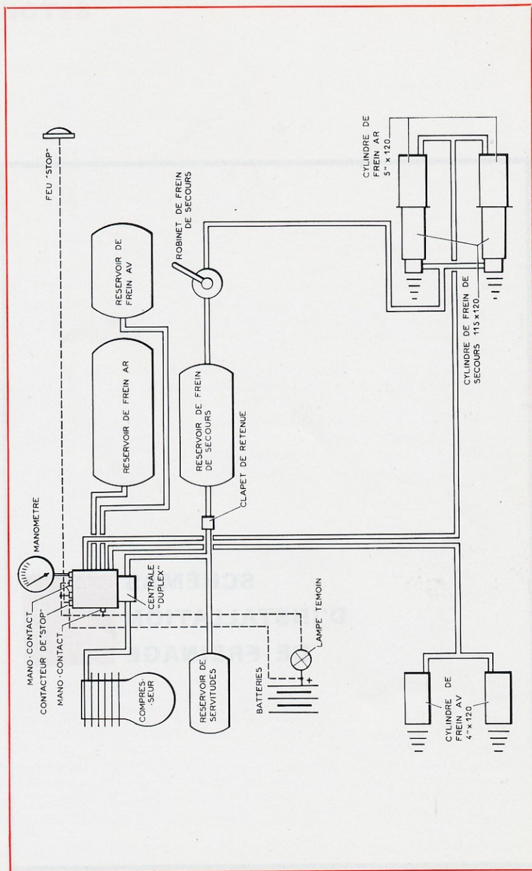
SCHEMA D'INSTALLATION DE FREINAGE (CENTRALE DUPLEX) CHASSIS VERCORS PORTEUR
