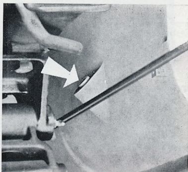
02-1 - Remplissage de la boîte de vitesses B 181.
