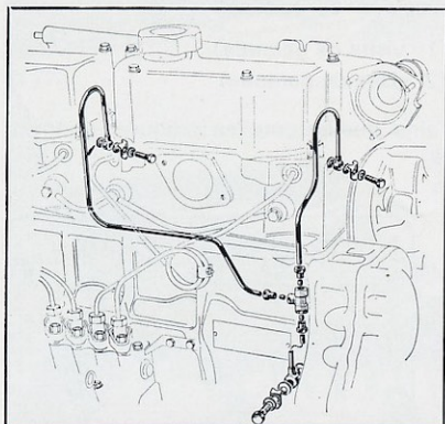
00-6 - Raccords d'arrivée d'huile sur culasse.
