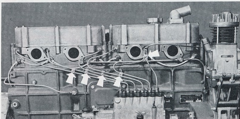
00-11 - Assemblage des tubes d'injection sur moteur 6 cylindres.
