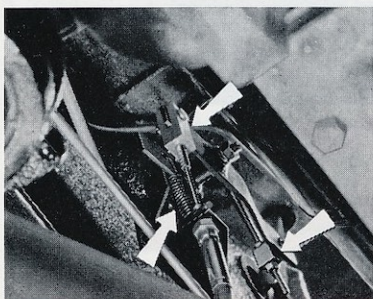
00-8 - Commande d'accélération C.S.A.
