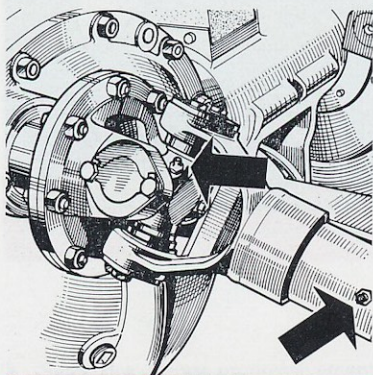
07-2 - Arbre entre pont AR et cardan véhicule 6 x 4.
