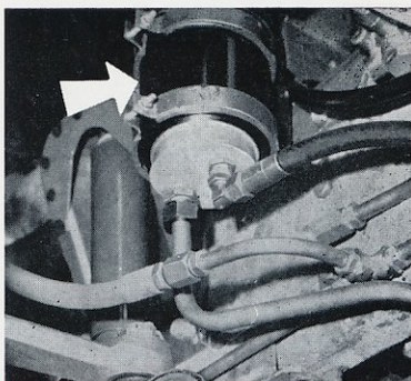
05-6 - Vidange du circuit hydraulique de servo-direction sur CA.
