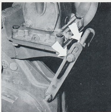
00-23 - Tension de courroie du compresseur.
