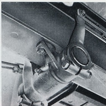
08-8 - Graissage chape côté extérieur sur renvoi intermédiaire de frein et graissage de l'axe sur (6 x 4).
