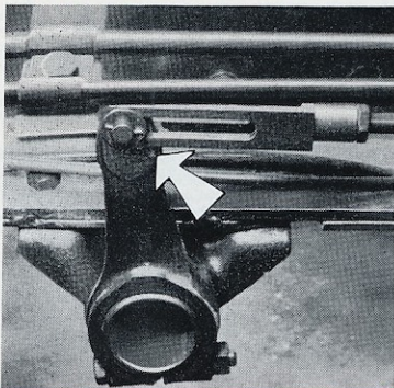
08-7 - Graissage chape côté intérieur sur renvoi intermédiaire de frein à main (6 x 4).
