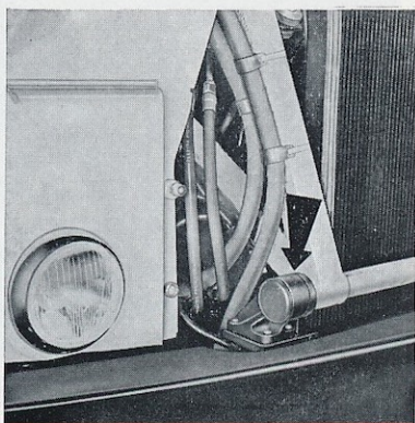
10-9 - Axes d'articulation de cabine.
