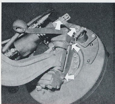
04-2 - Graissage axes de pivot - essieu E 251.
