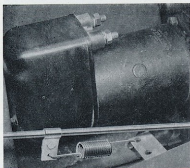
09-2 - Entretien du démarreur.
