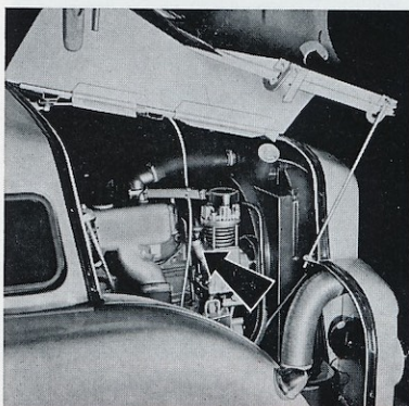
00-22 - Remplissage d'huile du compresseur sur CSA.
