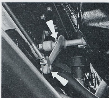
01-1 - Graissage de la Commande de débrayage CA ou CSA.
