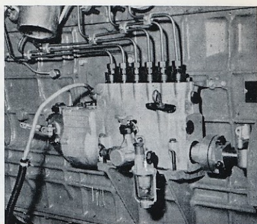
00-7 - Pompe d'injection 6 cylindres.
