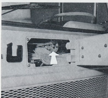
10-2 - Emplacement moteur essuie-glace - CA.
