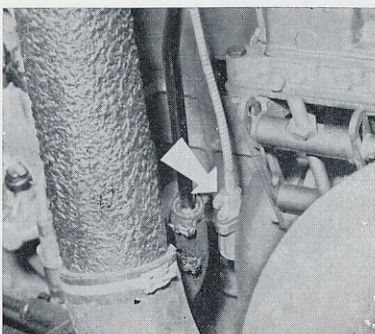
10-4 - Prise de compte-tour sur moteur
