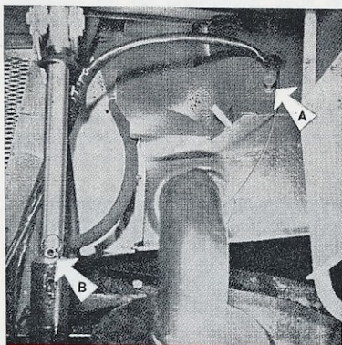
10-10 - Commande de démarreur sur cabine.
