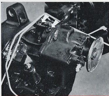
03-4 - Orifice de remplissage de carter principal et carter boîtier de différentiel sur Pont AR n° 1 (chassis 6 x 4).
