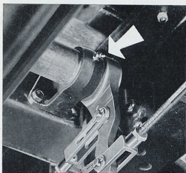
08-1 - Graissage axe de palonnier et chapes (6 x 2).
