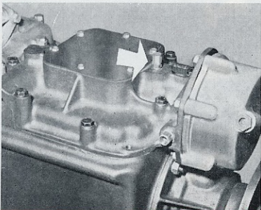
02-4 - Soupape d'aération sur boîte de vitesses B 181.
