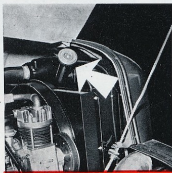
00-19 - Bouchon de remplissage du radiateur sur C.S.A.
